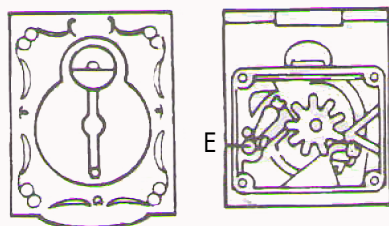
Монетоприемник (12)
